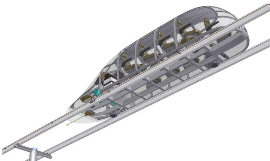
Рис. 5. Компоновка высокоскоростного юнибуса Ю-321РЕ (вид снизу)
