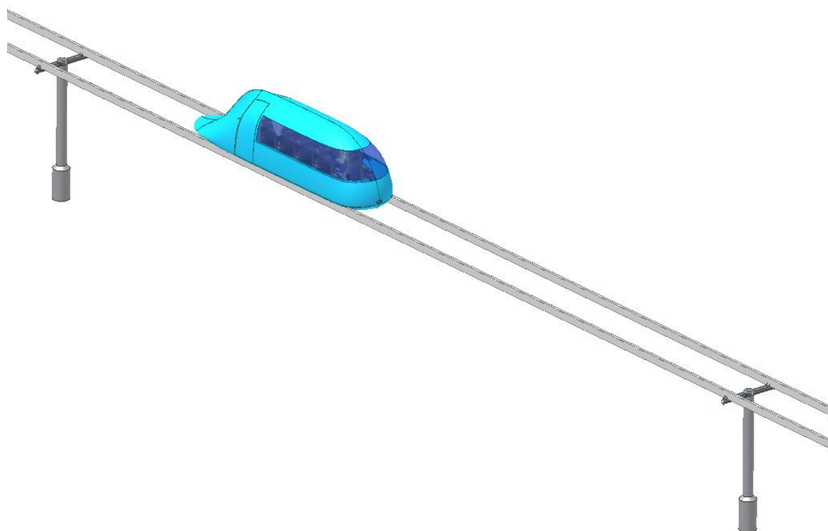
Рис. 1. Общий вид высокоскоростного юнибуса модели Ю-321РТ (вид сверху)
