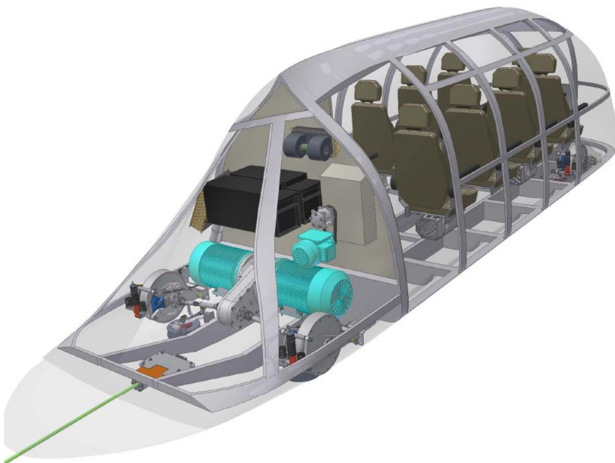
Рис. 4. Компоновка высокоскоростного юнибуса Ю-321РЕ (вид на корму)
