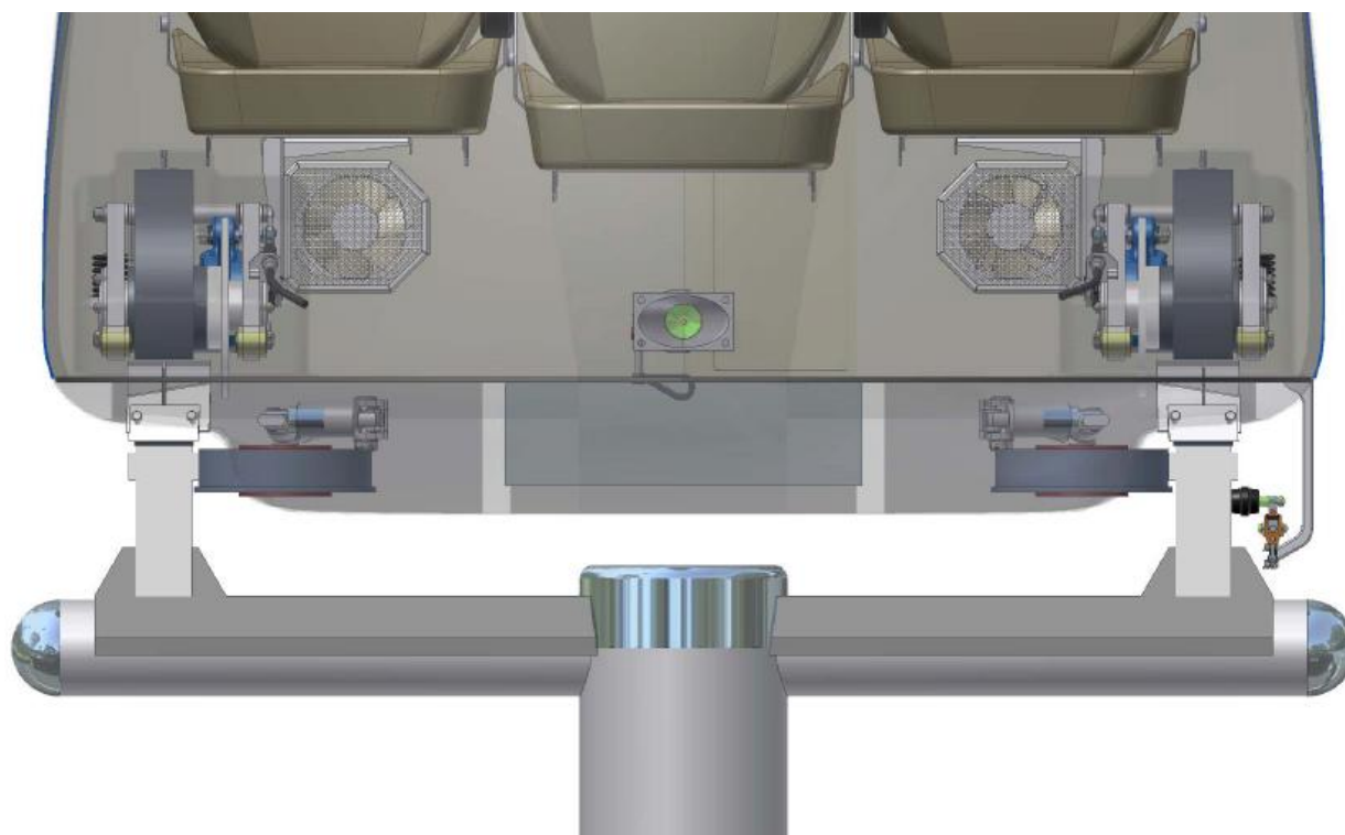
Рис. 7. Схема размещения направляющего и противосходного устройства юнибуса Ю-321РЕ (справа показан токосъем)
